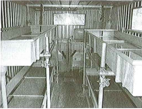
Fig. 2 - Piccolo incubatoio di valle (APDT).
